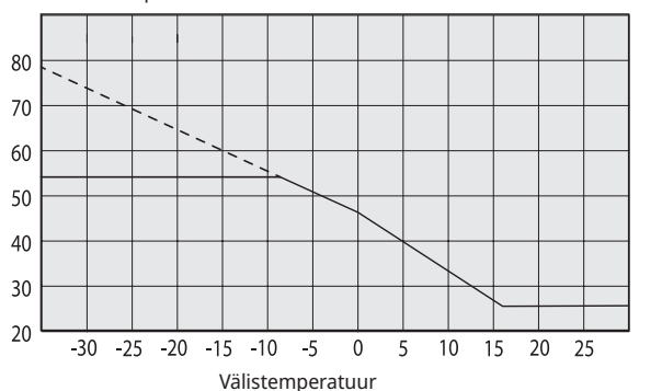
Pealevoolu temperatuur
