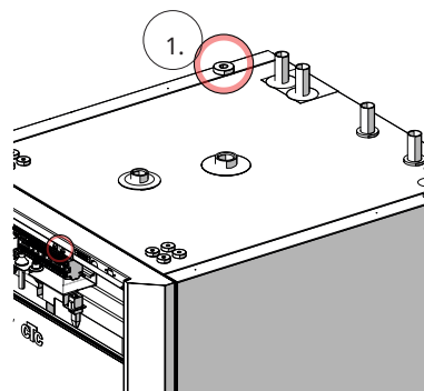
Toitekaabli paigutus.
