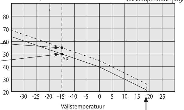
Pealevoolu temperatuur
