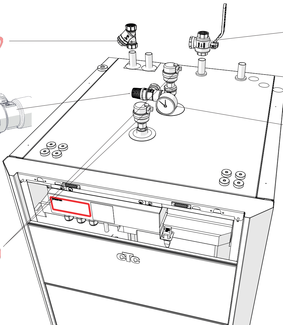
Ohutusventiil
