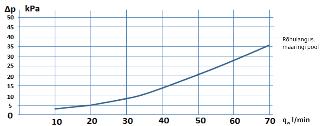
CTC GSi 616
